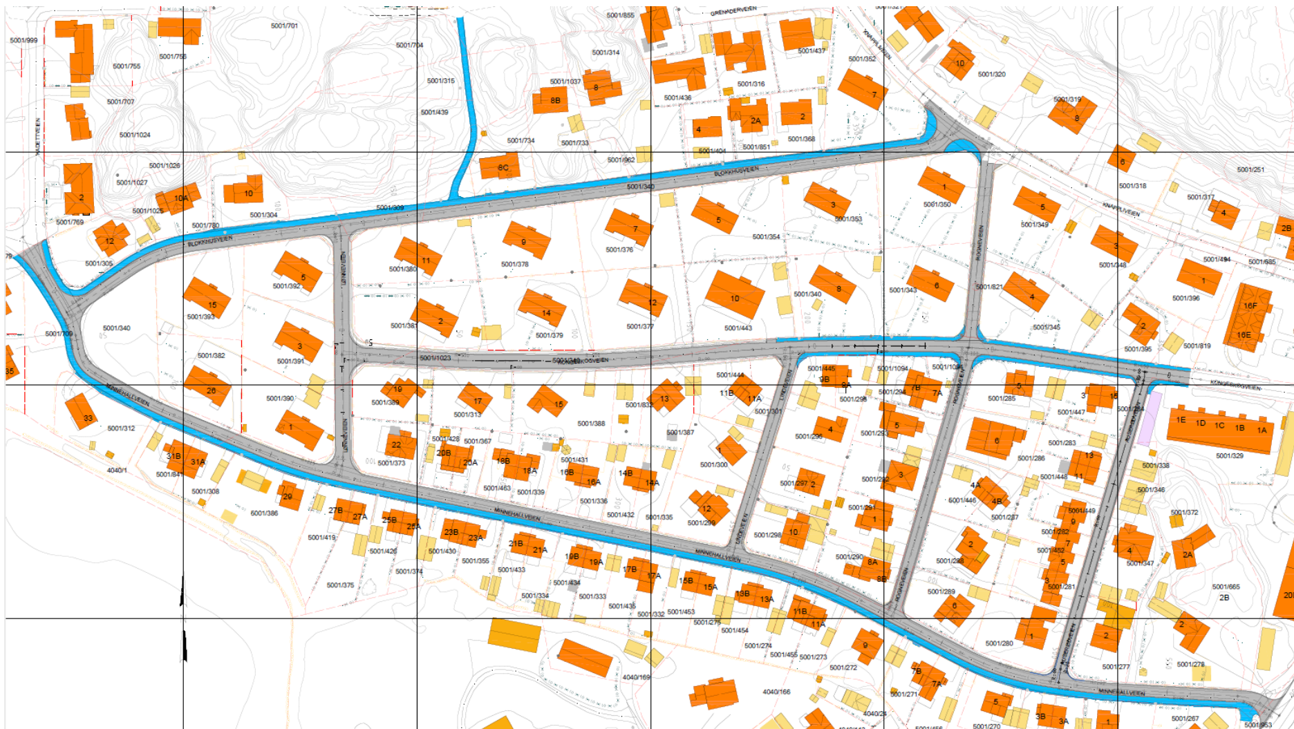
Figur 2 - Veiplan – oversikt over vei og fortaulsløsning
